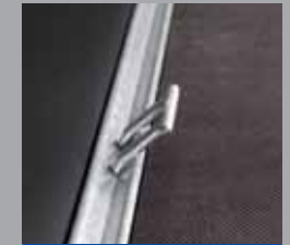
Anbindepunkte in V-Profil (Standard) DIN 400 daN (kg)
