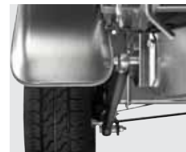
8 Stossdämpfersatz, gebremsten Modelle (Option)
